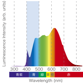
IXM シリーズに使用している超高演色 LED の発光スペクトル
